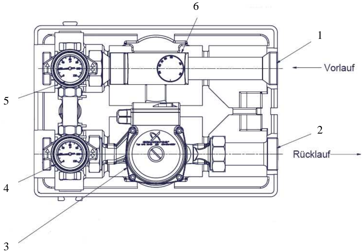
Abbildung 5.1: Anschlussgruppe
